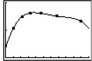
y = P_4(x)
