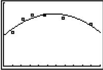
y = P_2(x)
